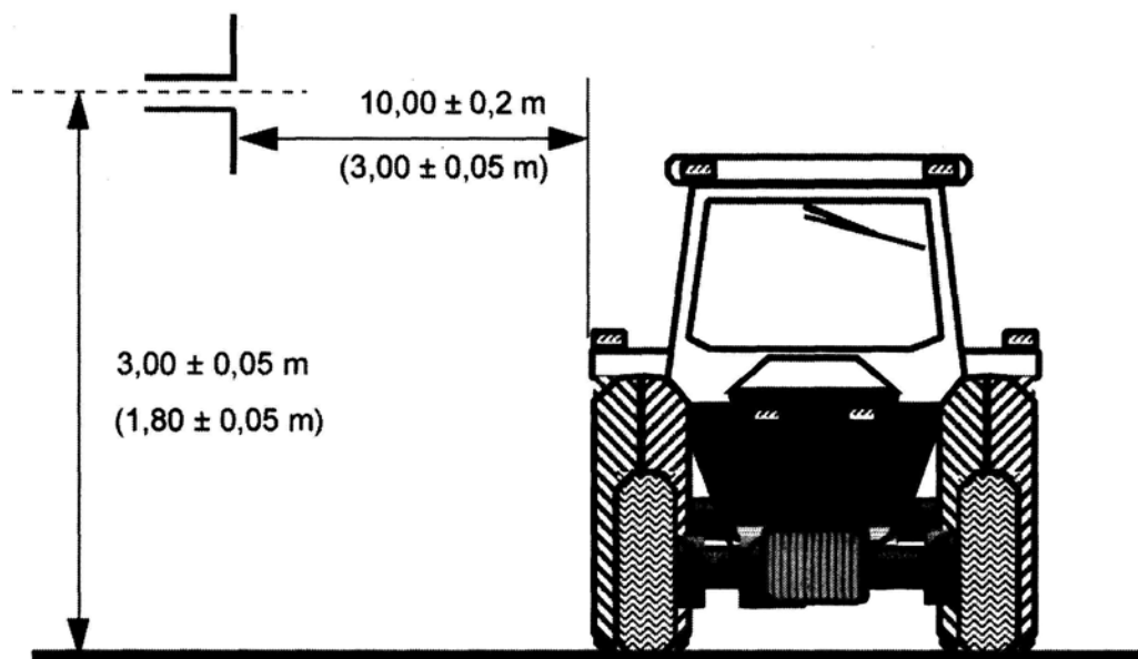
Elevation
