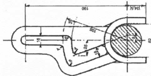
Celle de positionnement des portes-ameselles Keil zur Festlegung der Bremsklötze Stop-block for positioning brake-shoe holders
