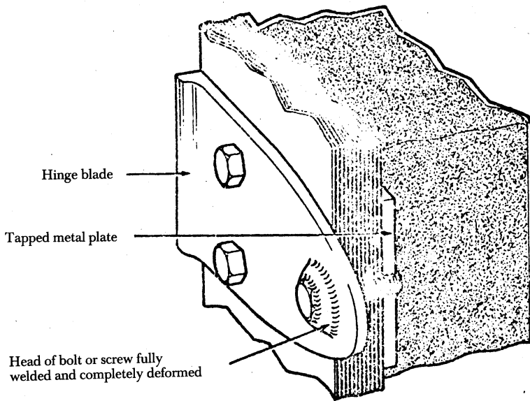
Hinge
